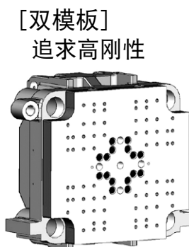
多型腔模具 薄壁成型品 等
